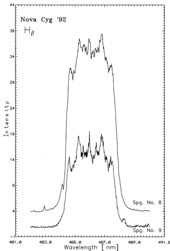
Abbildung 12.4: Ausschnitt eines hochauflösten optischen Spektrums mit einer verformten H \beta -Linie ( \lambda_0 = 486,1 \text{ nm} ). (T.L. Hayward et al. 1992).
